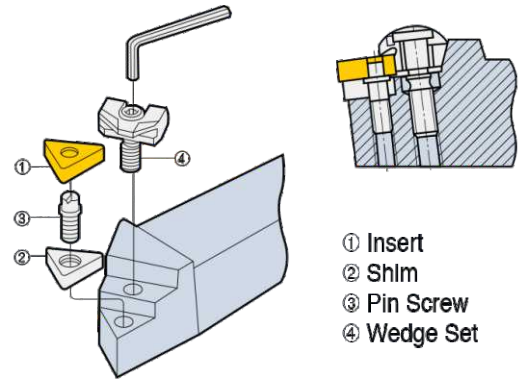
W-Wedge Clamp Type W型压紧方式
