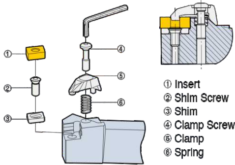
D-Clamp Type D型压紧方式
