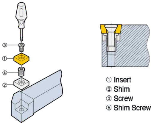
S-Screw Clamp Type S型压紧方式
