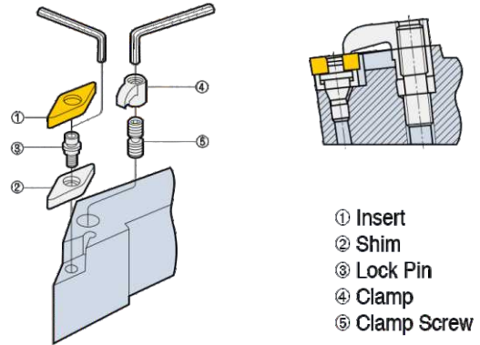
M-Multi Lock Type M型压紧方式
