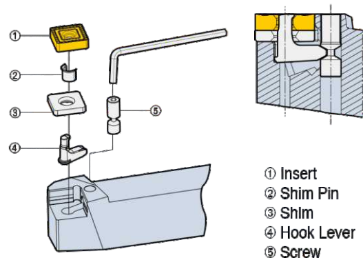
P-Lever Type P杠杆型压紧方式
