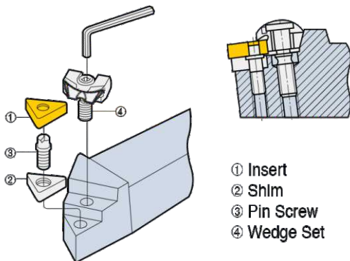
B-Clamp Holder B型压紧方式
